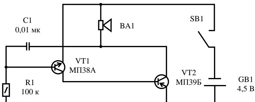
Рис.8.2. Схема звукового генератора
