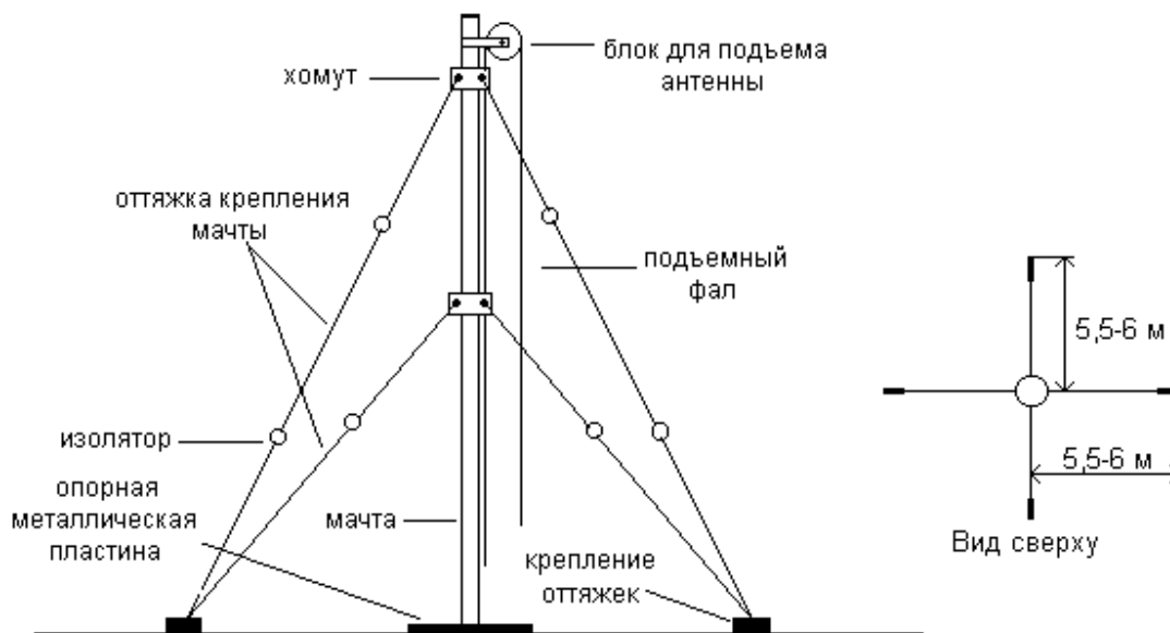
Рис.2.8. Антенная мачта в развернутом виде
